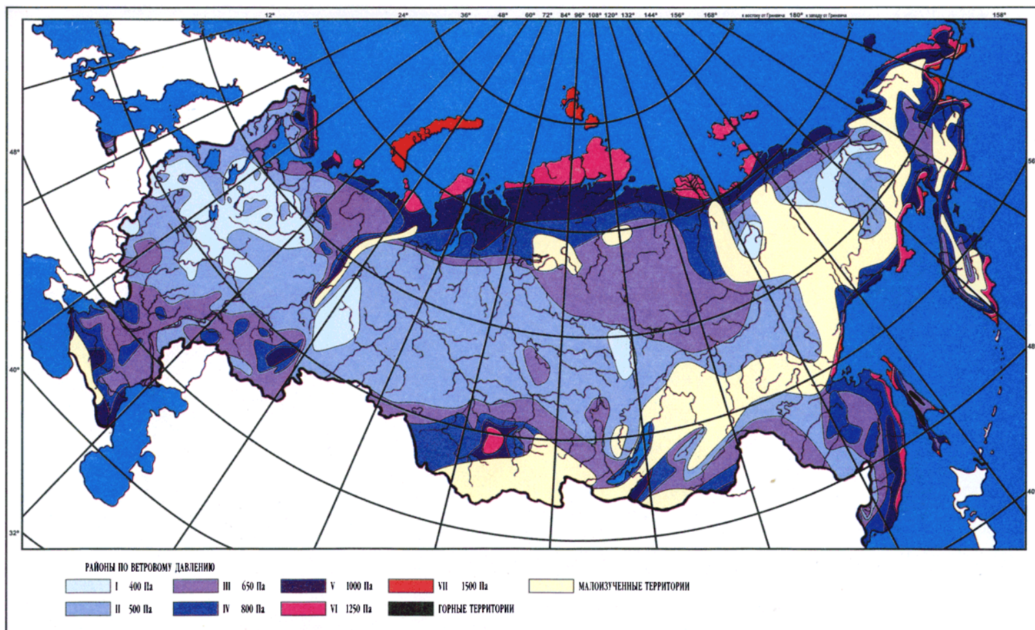
Рис.2.5.1. Карта районирования территории РФ по ветровому давлению
